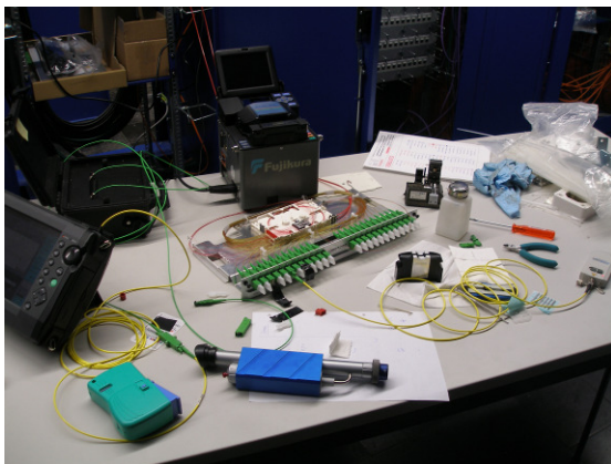
Spleiss- und Messarbeiten am Rack
