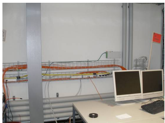
Messvorspann für die OTDR-Messungen
