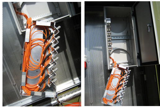
Steckmodule mit DIN-Schienen Halterung von Fiberswiss AG
