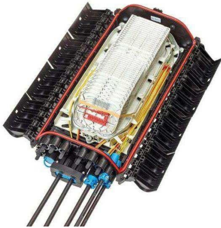
Wasserdichte (IP68) Spleißmuffe BPEO Evolution Size 3 (Grösse 3)
